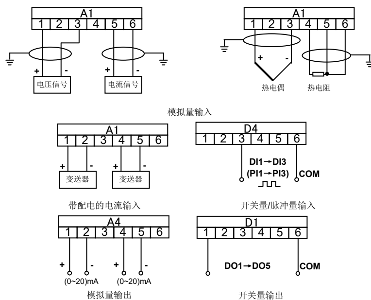
图 2-6 信号线的连接
