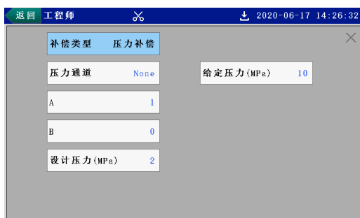
图 8-6 线性压力补偿画面
