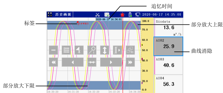
图 10-2 历史画面
