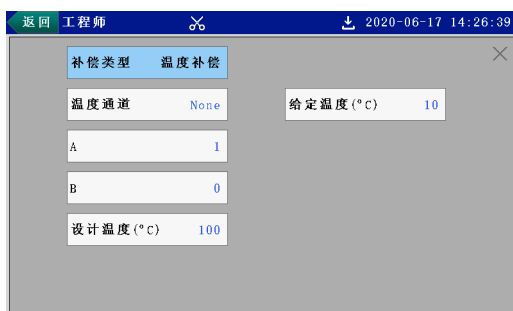
图 8-7 线性温度补偿画面
