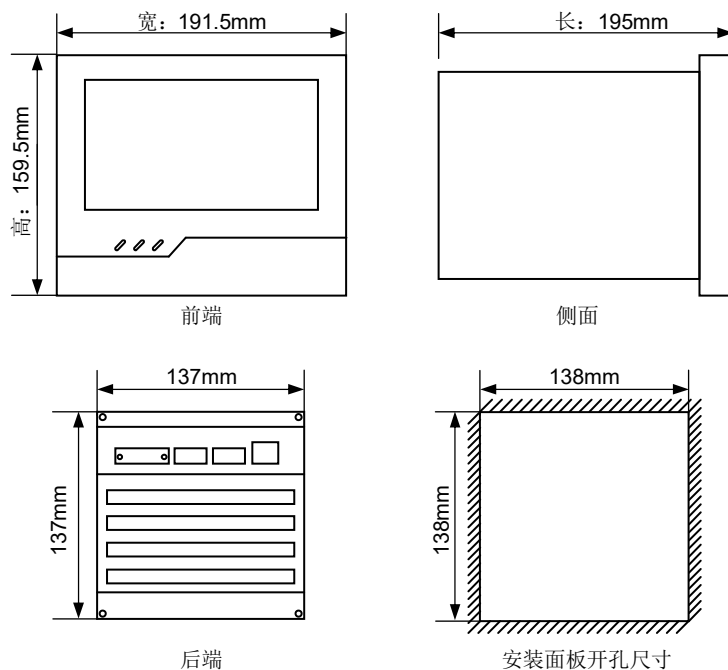
图 2-2 安装尺寸
