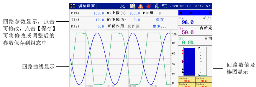
图 6-3 PID 调整画面
